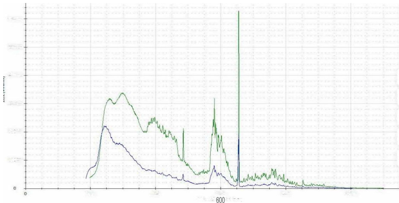
ATP5200 -----; ATP520R ----- Спектры излучения ртутно-аргоновой лампы, зарегистрированные спектрометрами при одинаковых условиях измерения
