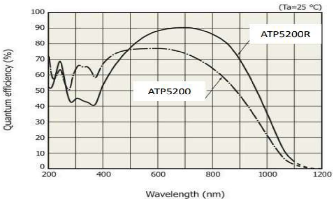
ATP5200 и ATP5200R спектрометр – фотометрическая чувствительность детекторов
